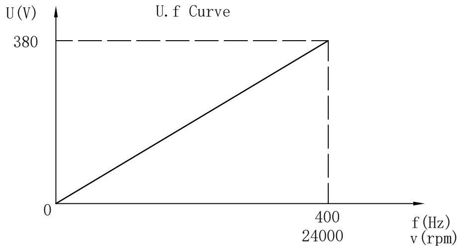
频压曲线
